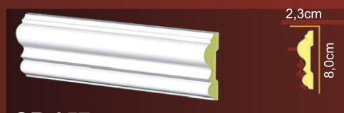
GR 057 - Barra de 2,20m
